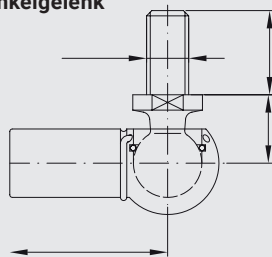
Winkelgelenk
